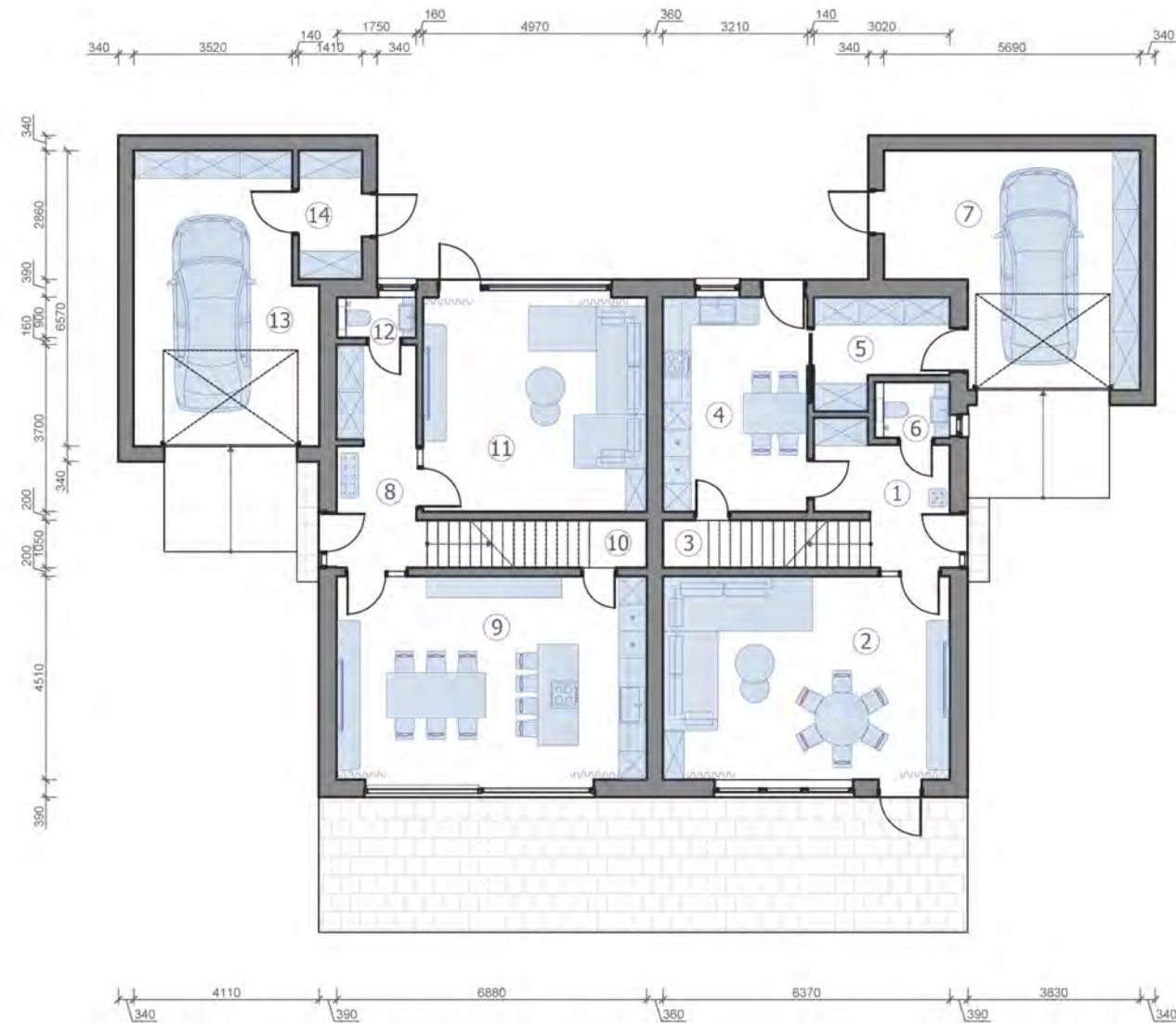
Grundriss 1. 1:100 (A-3)
