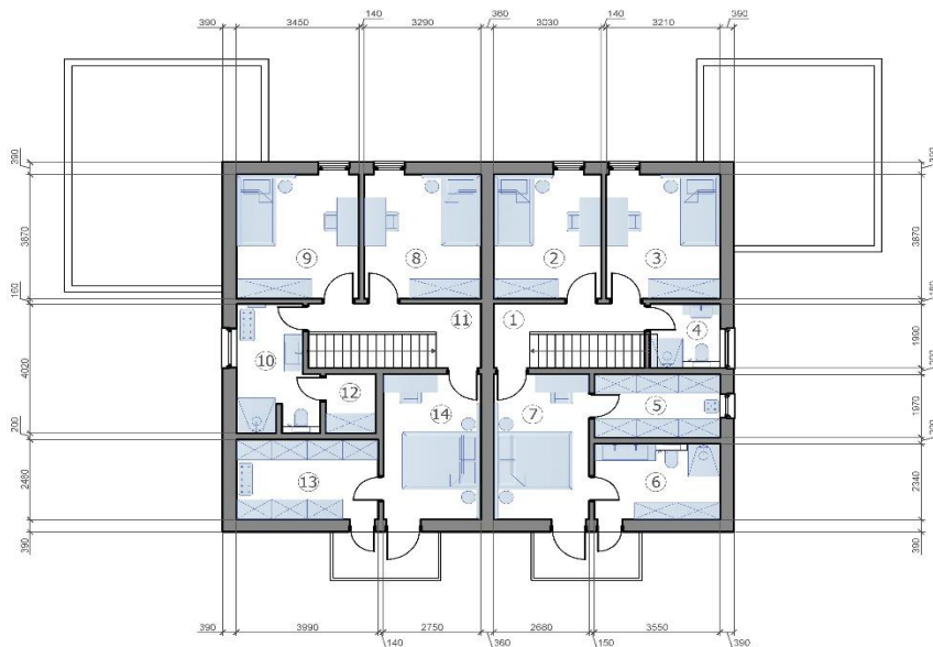
Grundriss 2. 1:100 (A-3)
