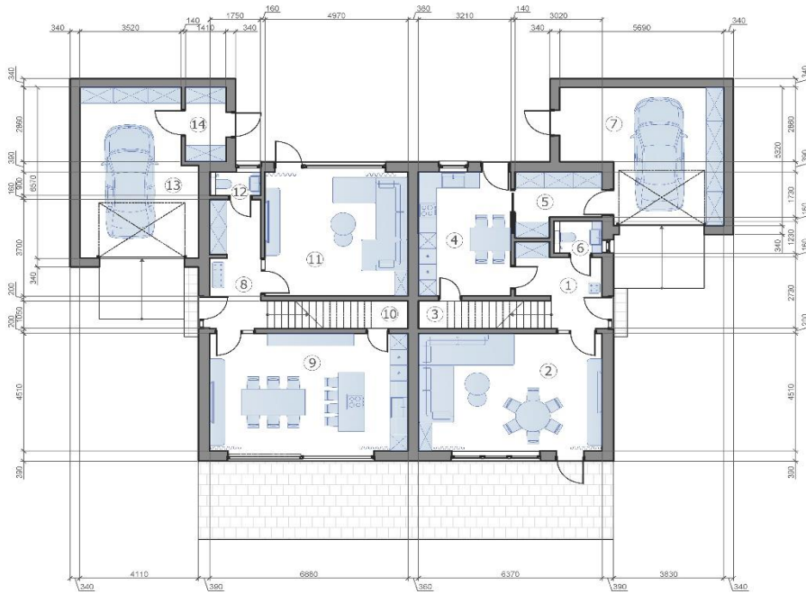
Grundriss 1. 1:100 (A-3)
